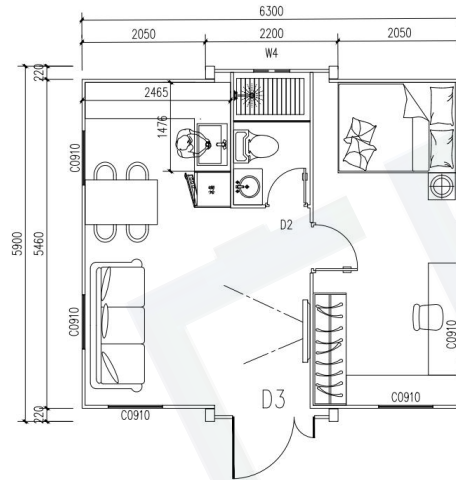
20ft - 1 bedroom
