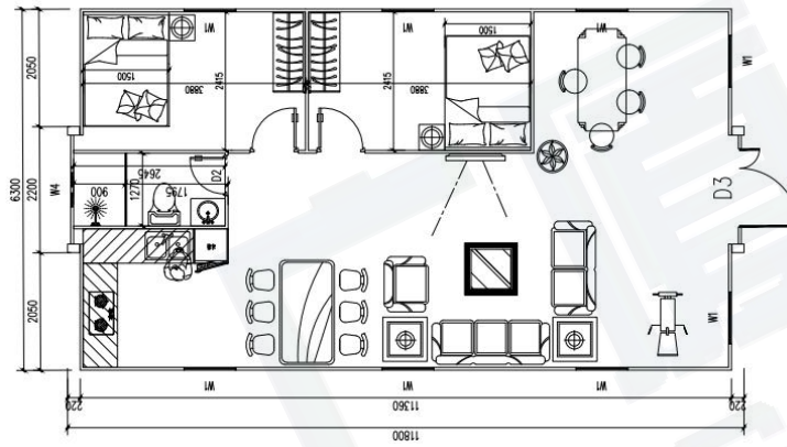
40ft - 2 bedroom
