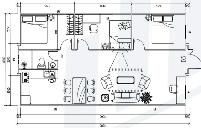
40ft - 3 bedroom
